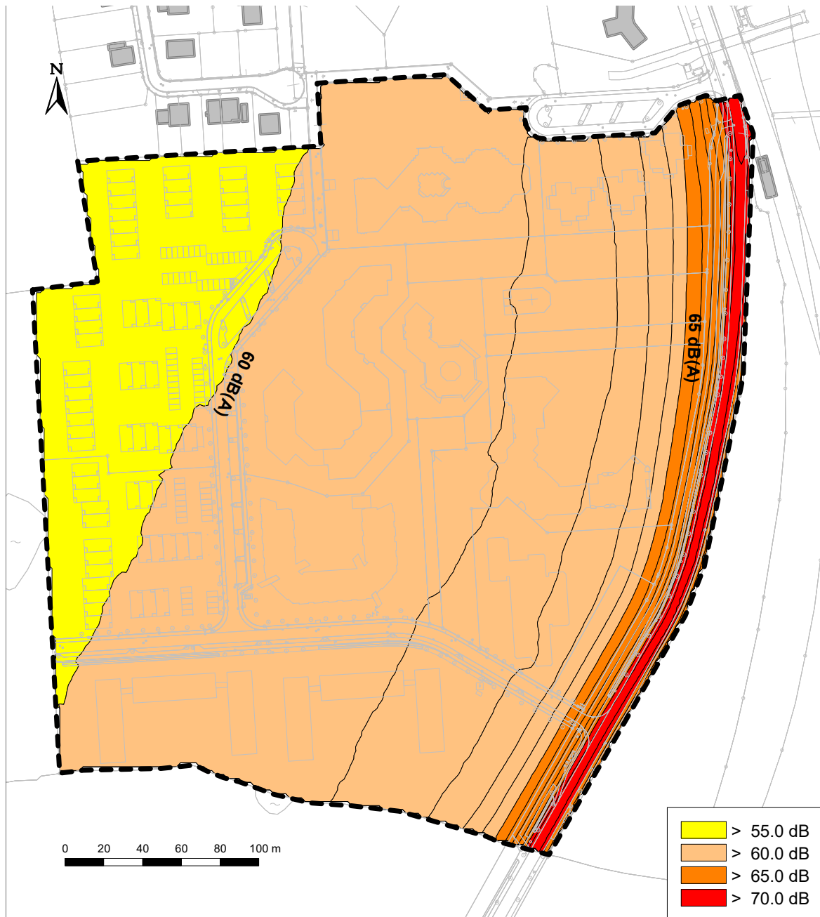
Abbildung 1: maßgeblicher Außenlärmpegel für schutzbedürftige Räume, Maßstab 1:2.500
