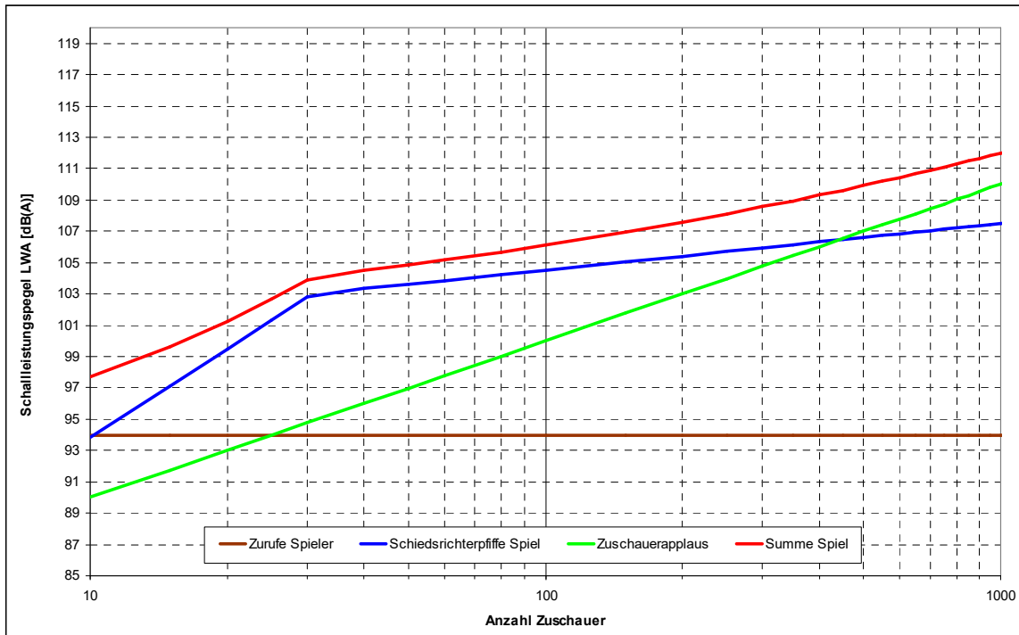
Abbildung 1: Schalleistungspegel beim Fußball in Abhängigkeit von der Anzahl der Zuschauer [14]
